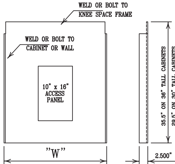
BACK ENCLOSURE PANEL — OPTIONAL —
